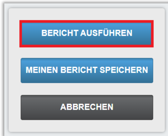
Abbildung 6 - Bericht ausführen
