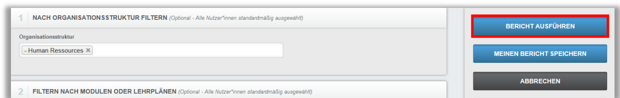
Abbildung 10 – Bericht ausführen
