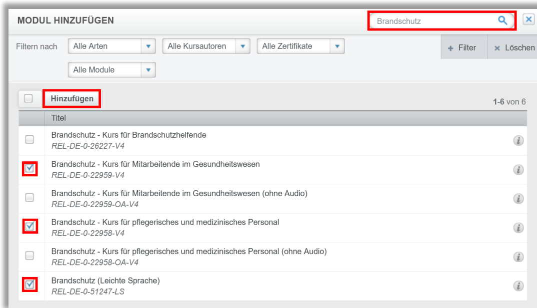
Abbildung 5 – Modul hinzufügen
