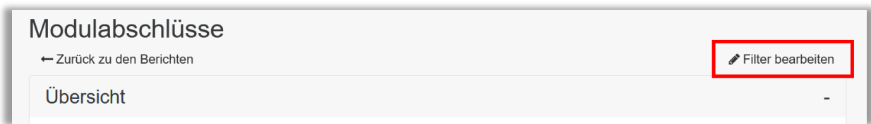
Abbildung 14 – Filter bearbeiten
