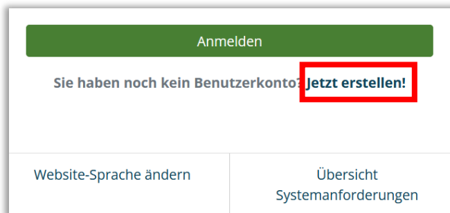
Abbildung 3 – Registrierungsformular aufrufen
