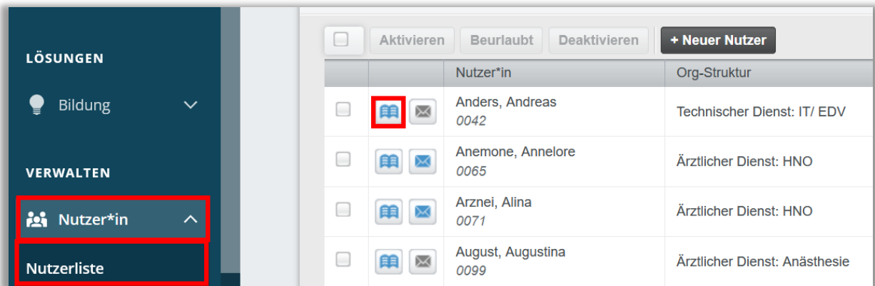
Abbildung 4 - Leistungsnachweis aufrufen
