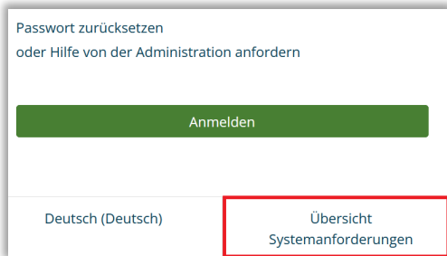
Abbildung 10 –Systemanforderungen
