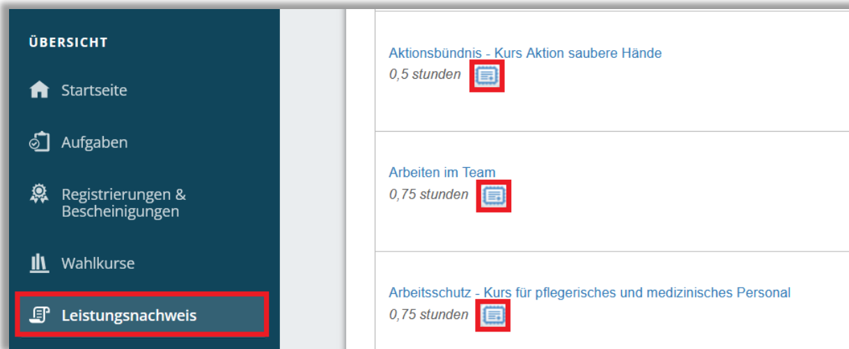
Abbildung 13 –Zertifikate
